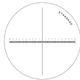
No. S-100 メモリ幅 20mm 0.1mm 間隔 外径φ26 厚み t1.3
